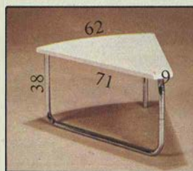
GRAD. Trekantigt kombinationsbord. (45°). Mått: 71x62/9 cm, höjd 38 cm. Skiva: Vit plastfärg. Underrede: Förkromade rör. Monterbart. Vikt 9 kg. Krom/vitlack kr ..... 98:–
